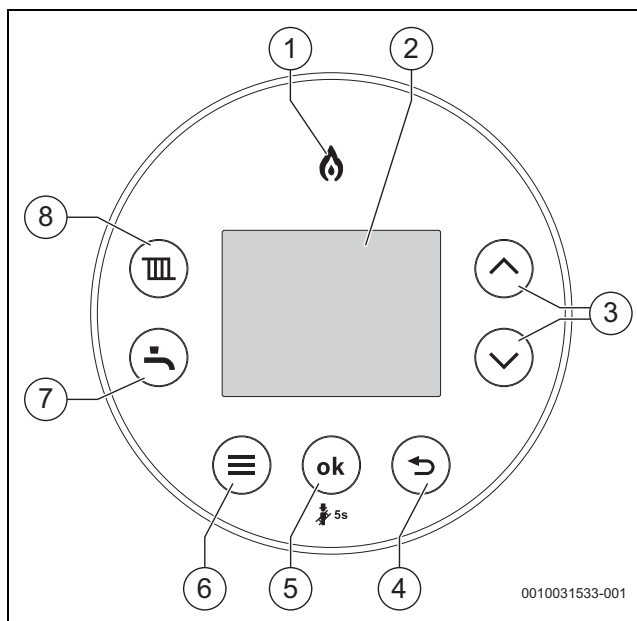
Obr. 2 Ovládací panel
