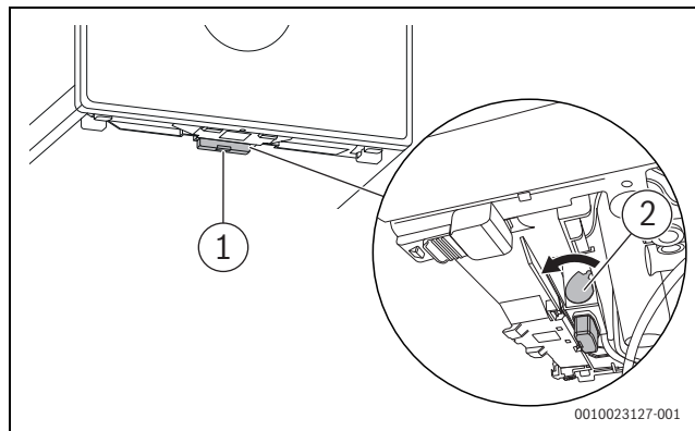
Obr. 4 Zajištění Key
