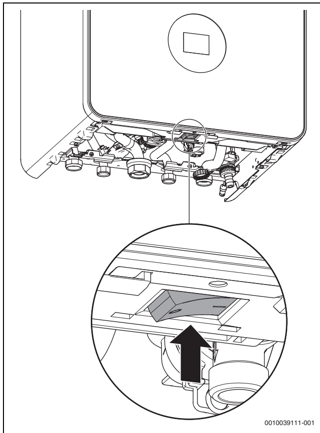
Obr. 1 Hlavní vypínač
